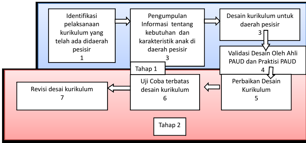
Gambar 1. Langkah penelitian
